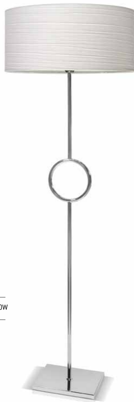
034/P CROMO COR 527 Ø 27x20 cm H 138 cm 1 x E27 / 60W 45x45x25 cm H 154 cm
